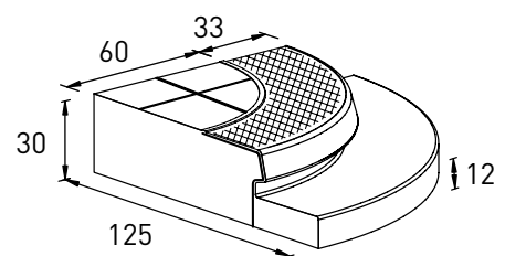
Hoekstuk 18/20
