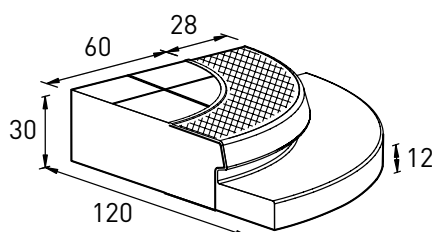
Hoekstuk 13/15
