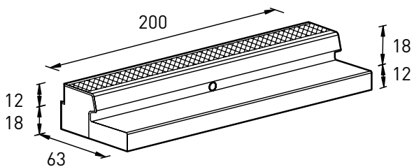
Doorsnede - Busperronband 13/15
