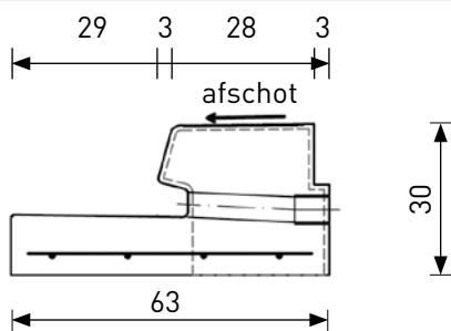
Overgangsbands 13/15 - links/rechts
